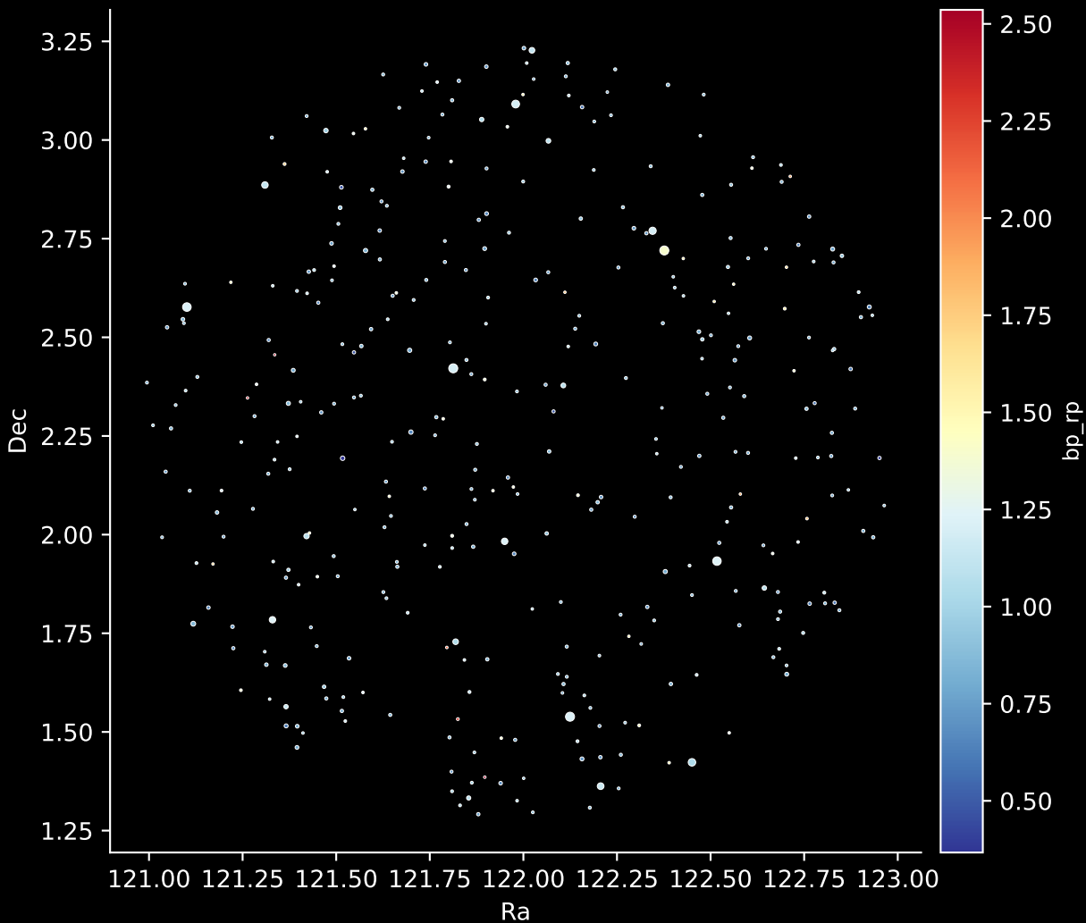
GALAH DR4 Field: [6681] Stars: 369
