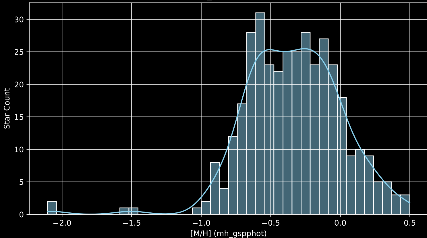
GALAH DR4 Field: [6681] [M/H] (mh_gspphot) (n= 365)
