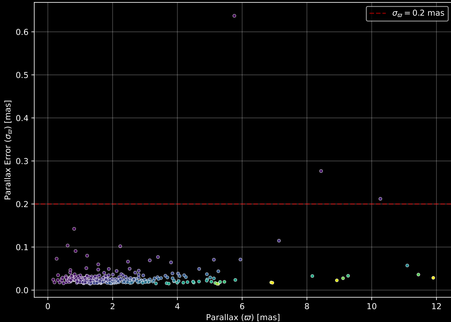
GALAH DR4 Field: [6681] Parallax Quality (n= 369)
